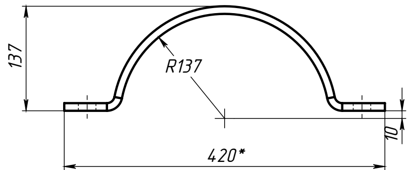
Поз.4 (Полухомут)
